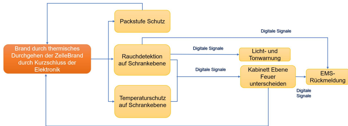
Logik der Feuerleitanlage
