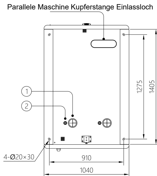
Schema der Installationsbohrung (Einheit: mm)
