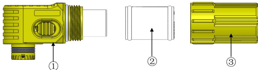
Terminal-Baugruppe Beschreibung
